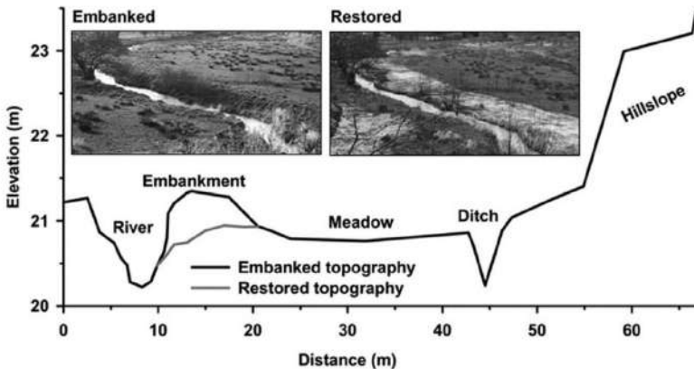
Gambar 7.2. Contoh pelaksanaan restorasi tanggul Sumber : Clilverd et al. , 2016
