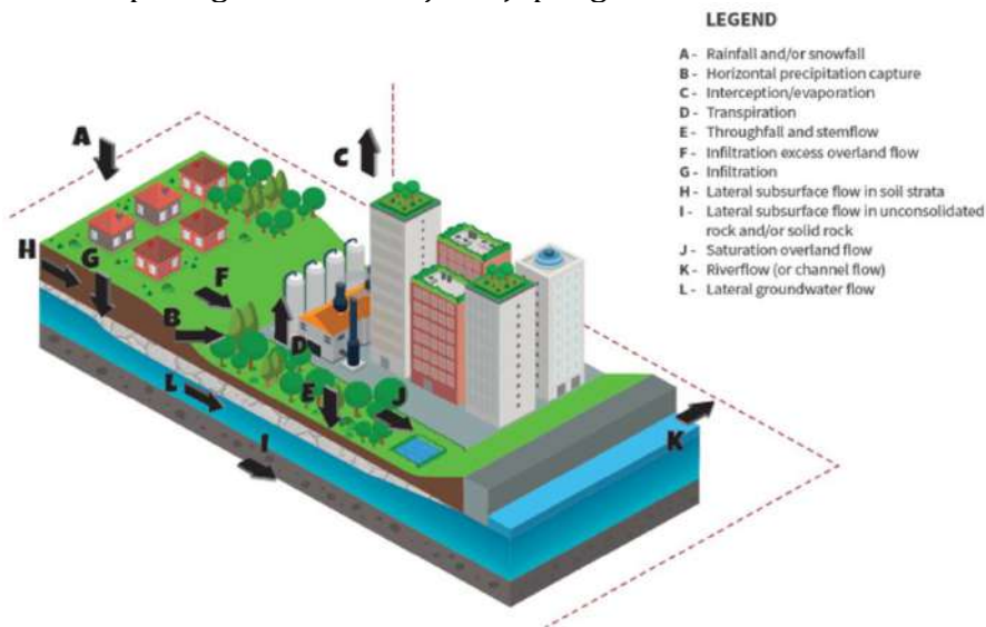
Gambar 5.11. Infrastruktur dalam manajemen banjir (Sumber : Meliala, L, 2024)
