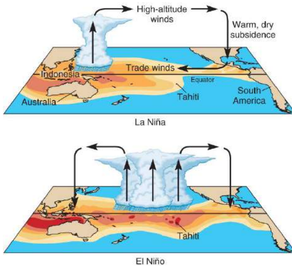
Gambar 5.10. Fenomena La Nina dan El Nino
