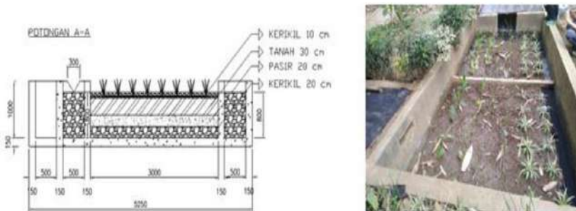
Gambar 7.5. Sistem lahan basah buatan
