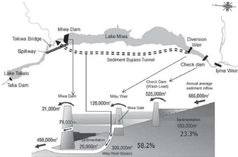
Gambar 7.4. Pengelolaan sedimen di reservoir menggunakan sistem sedimen bypass Sumber : Kondolf et al. , 2014
