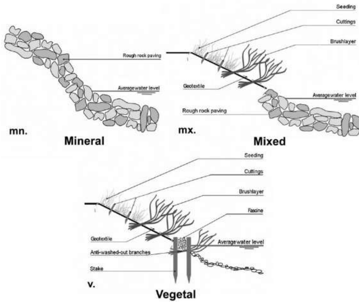
Gambar 7.1. Biorekayasa untuk Stabilisasi Tebing Sumber : Cavaillé et al., 2015
