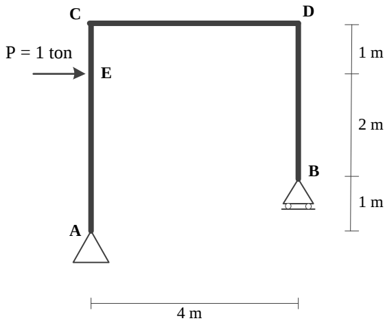
Gambar 10.7. Struktur Statis Tentu Kolom Tinggi Sebelah Dengan Beban Terpusat Horizontal Tidak Simetris
