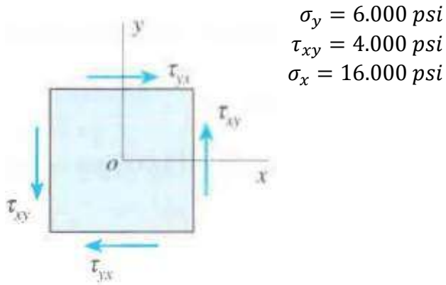
Gambar 7.18. Elemen yang berada dalam keadaan tegangan bidang
