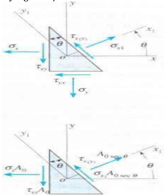
Gambar 7.15. Elemen tegangan dalam keadaan tegangan bidang: (a) tegangan-tegangan yang bekerja di elemen, dan (b) gaya-gaya yang bekerja di elemen tersebut
