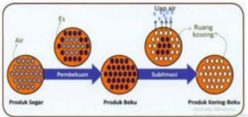
Gambar 4.3. Gambaran Prinsip Pengeringan Beku ( Freeze Drying )
