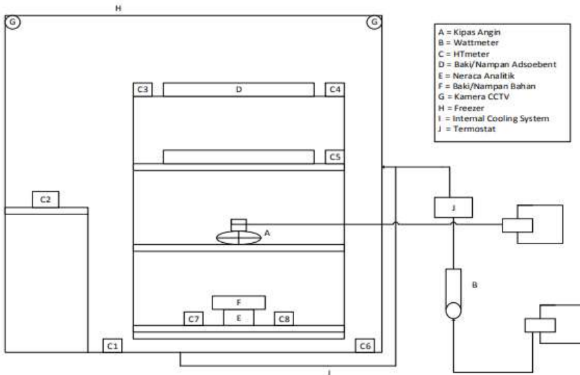
Gambar 4.5. Skema Pengeringan Dengan Closed Loop Drying
